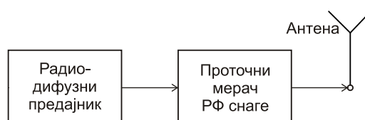
Слика 6.5-1 – Блок шема повезивања мерних инструмената
